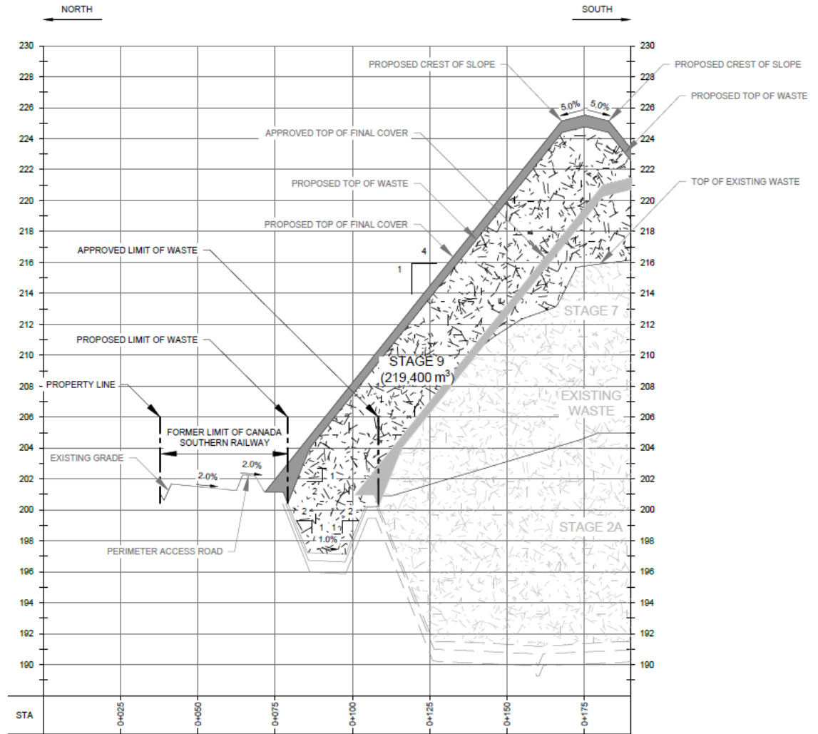
SECTION A-A' H=1:1000, V=1:200 CI-101
